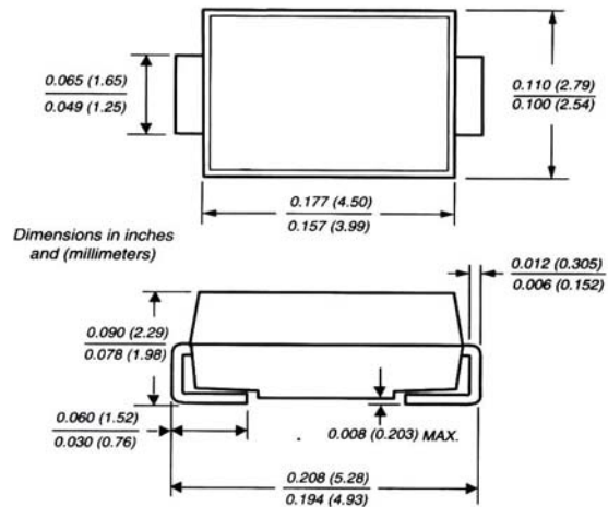
DO-214AC (SMA)
